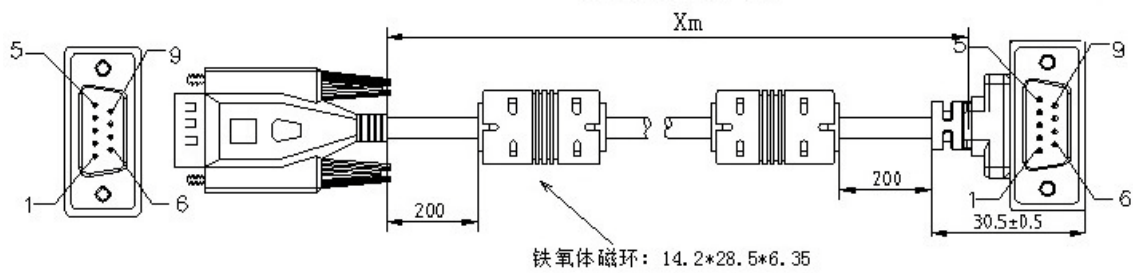
图AA.4 ZGCHDB9M-B-Xm连接器外形尺寸
