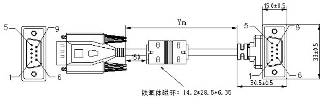
图AA.5 ZGCHDB9M-B-Ym连接器外形尺寸
