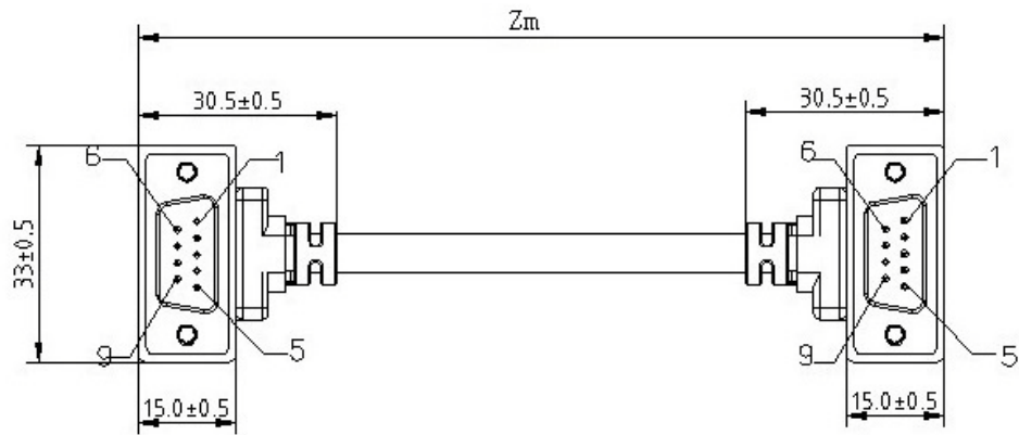
图AA.3 ZGCHDB9M-A-Zm连接器外形尺寸
